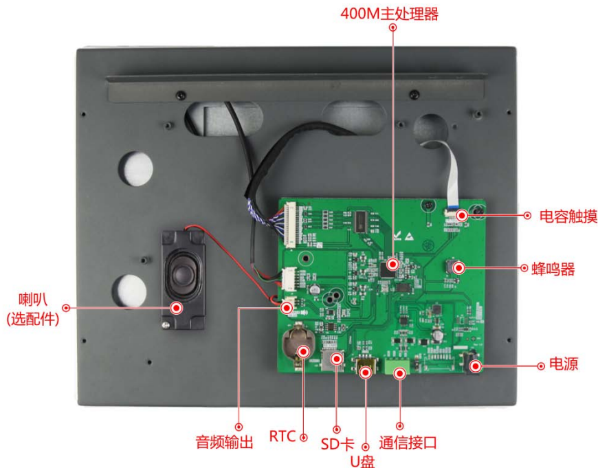
图 1-2 硬件配置图
