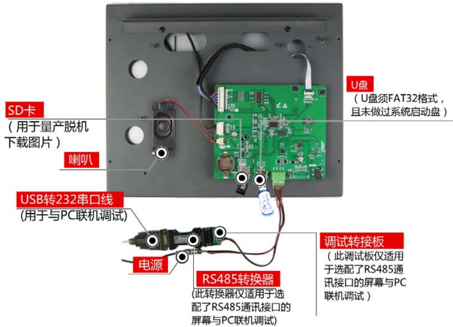
图 1-3 RS485 调试工具图
